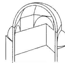
Klostergewölbe auf Trompen
